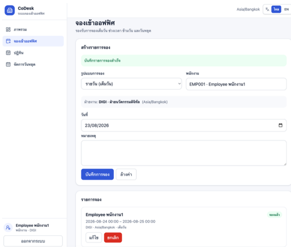
รูปที่ 4.1 การบันทึกรายการจองเข้าออฟฟิศสำเร็จ
