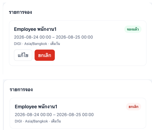
รูปที่ 4.12 การยกเลิกการจอง (ก) ก่อนยกเลิก (ข) หลังยกเลิก
